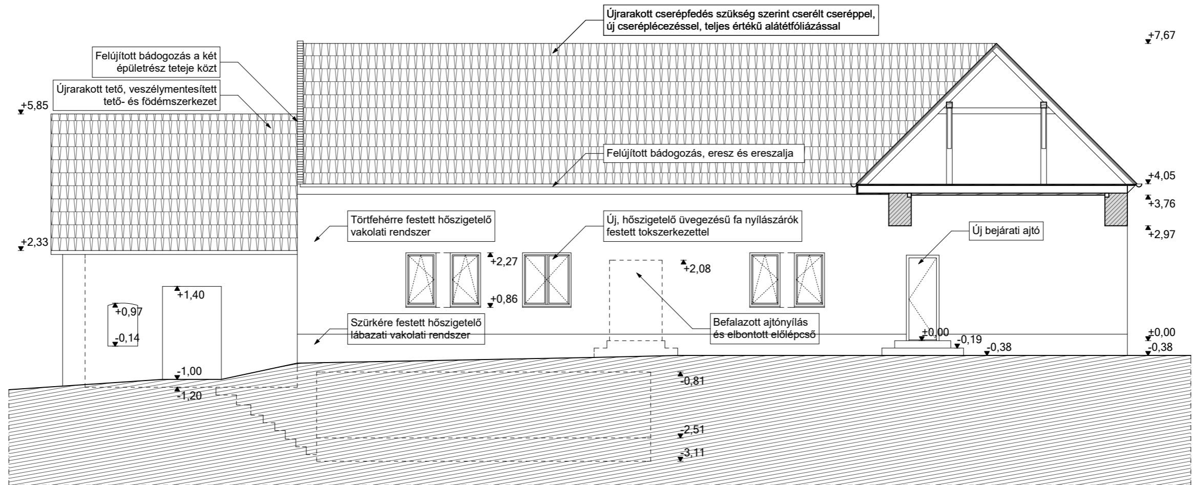
KELETI HOMLOKZAT
