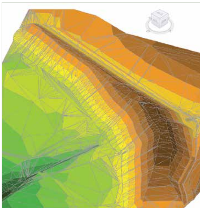
Hulladéklerakó rendezett térszín 3D modellje (részlet) - tervező: Golder-MKM konzorcium
