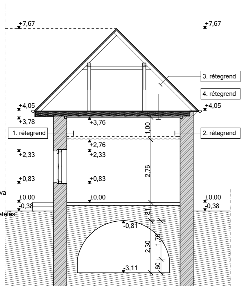
KERESZTMETSZET
