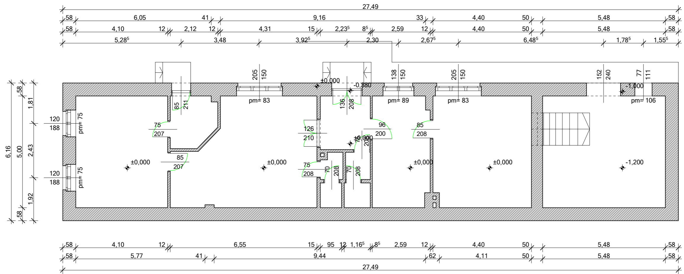
FÖLDSZINT FELMÉRÉSI ALAPRAJZA
